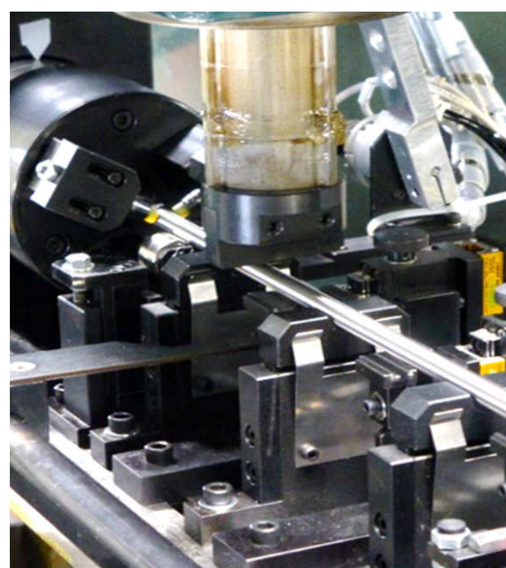
矯正装置
